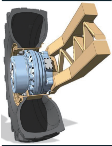
英国奎奈蒂克公司的轮内电动机 毂驱动技术
