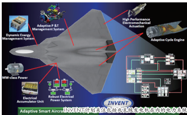
Adaptive Smart Aircraft INVENT计划关注包括兆瓦级发电机在内的电力系统
