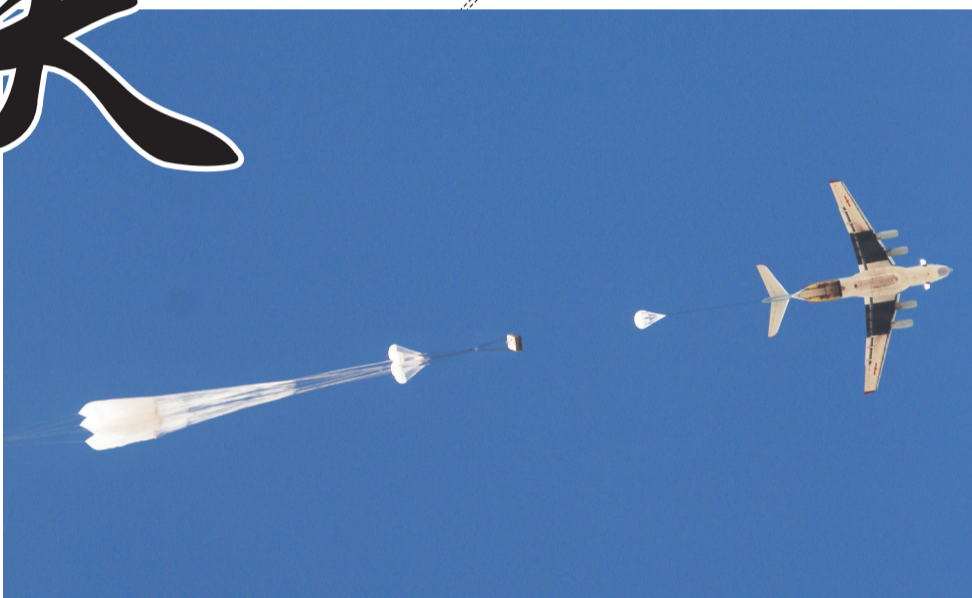
航空工业宏光：重装空投项目正在进行现场投放。 张笑然 摄
